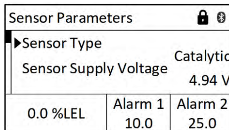
Figur 52 Eksempel på Sensorparametre-vinduet på hovedskærmen
