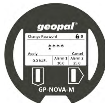
Figur 24 Brug af knapper til at vælge alfanumerisk tegn
