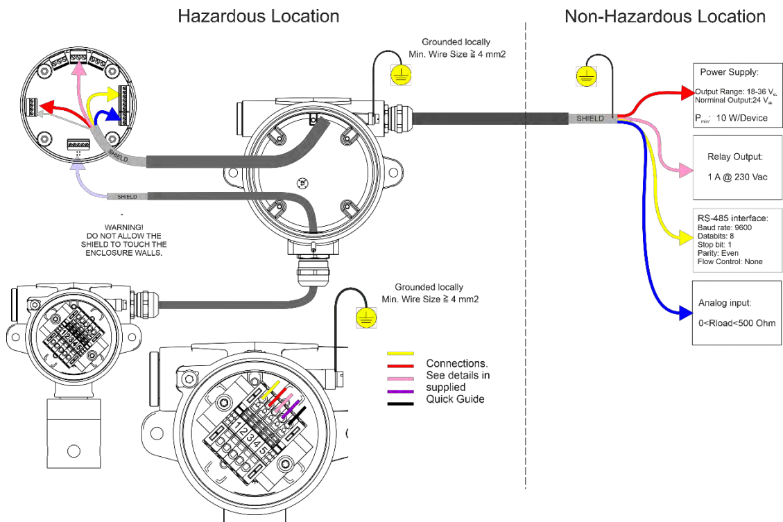
Figur 61 GP-NOVA-M og GJ-EX kabelføring
