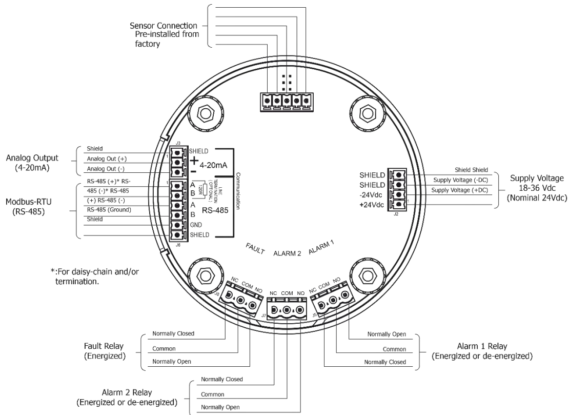
Figur 8 Forbindelsesterminaler til input board
