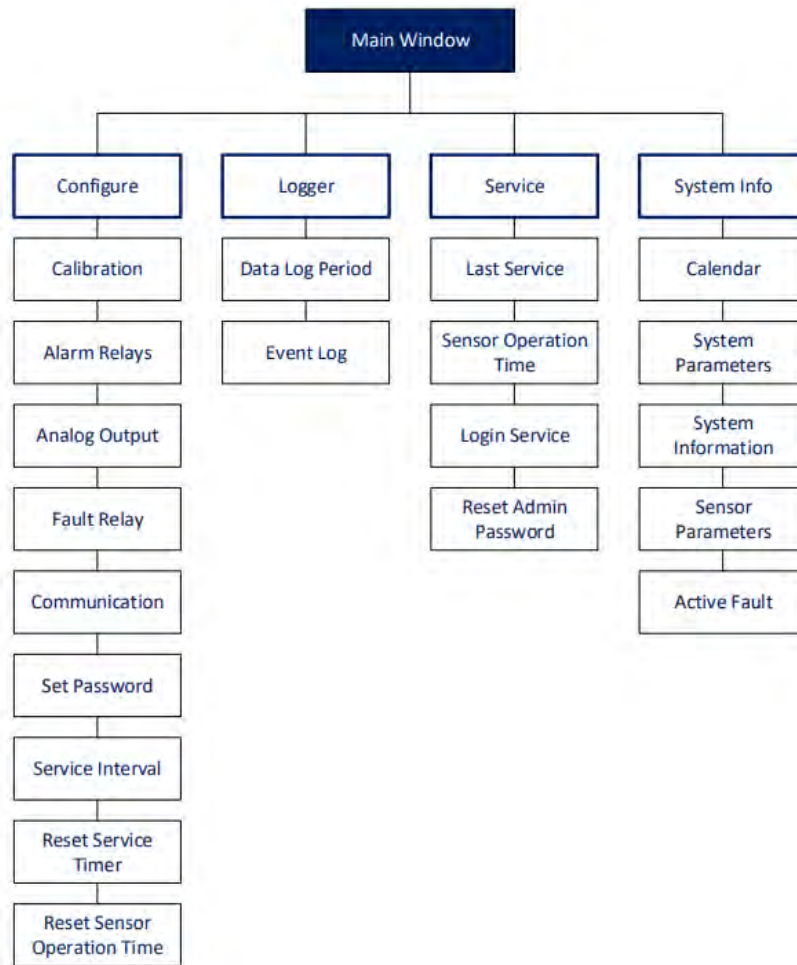
Figur 21 GP-NOVA-M menu struktur
