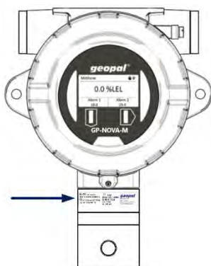
Figur 3 Etiketteplacering for sensor tryksikret kapsling
